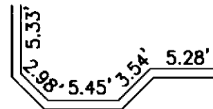
TYPICAL BAY WINDOW (D)
